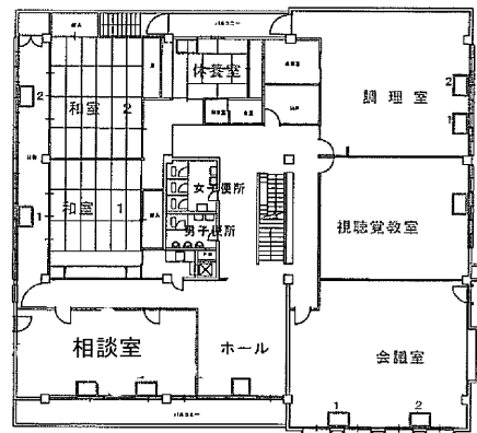
3 階
