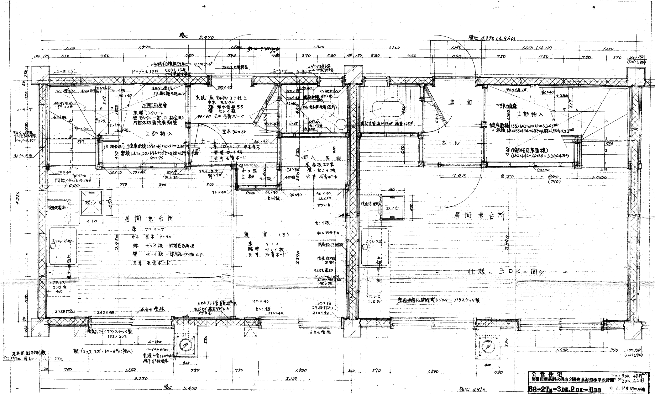
3LDK 1階平面 床面積 23.08㎡ (6.981坪)
