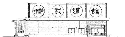
立面図 S-1/300
