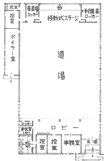
平面図 S-1/300
