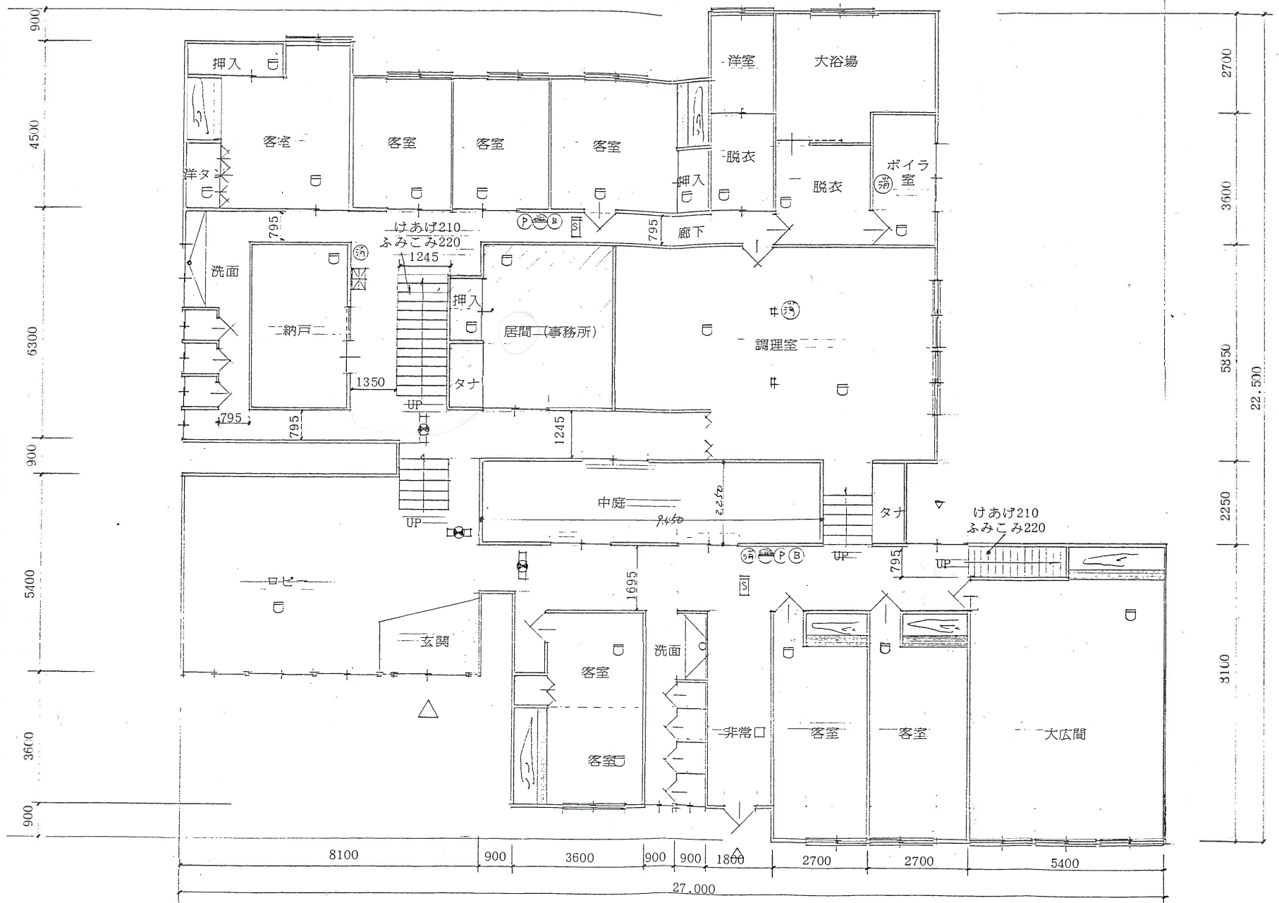
1階平面図 1:100
